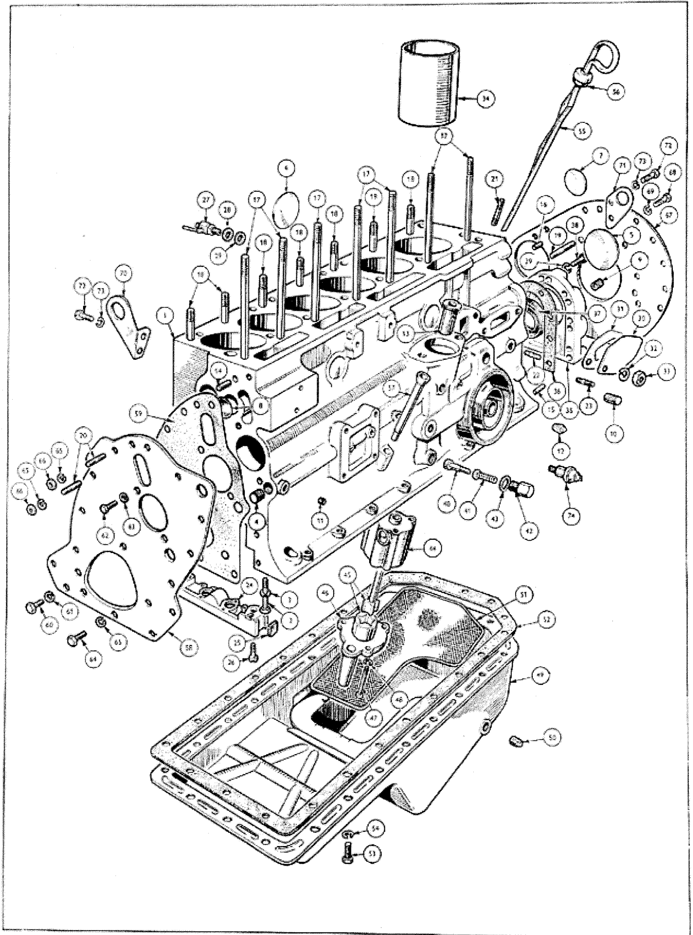
Moteur GT6 MK1
